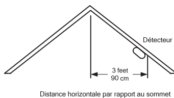
Figure 4 : emplacement d'installation recommandé pour les détecteurs de fumée et de chaleur dans des pièces munies de toits à pignon ou inclinés (pente > 20 degrés).
